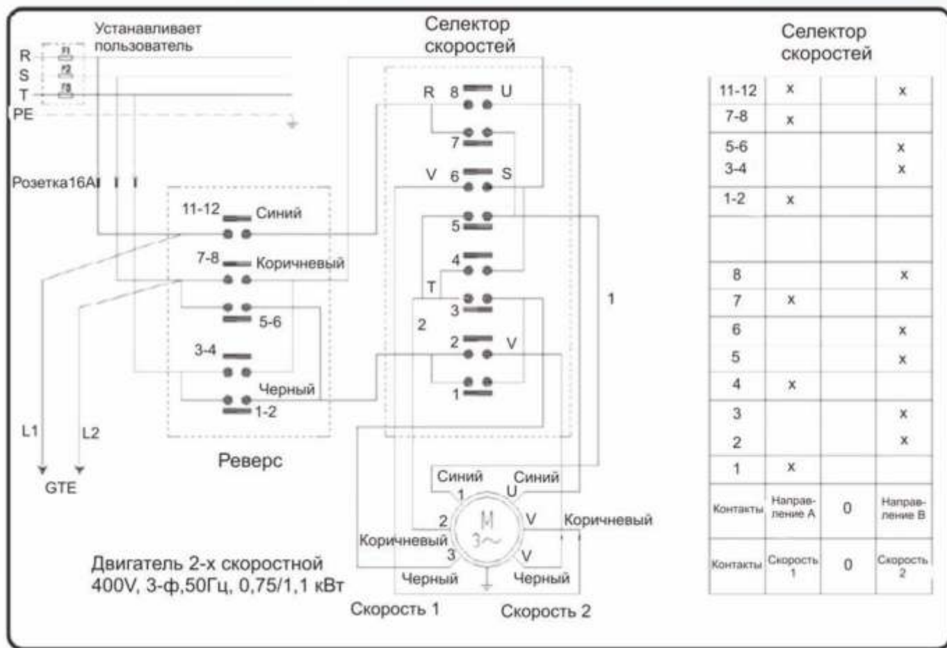
Электрическая схема, 230/400 В, 3-ф. двигатель, 2-хскоростной
