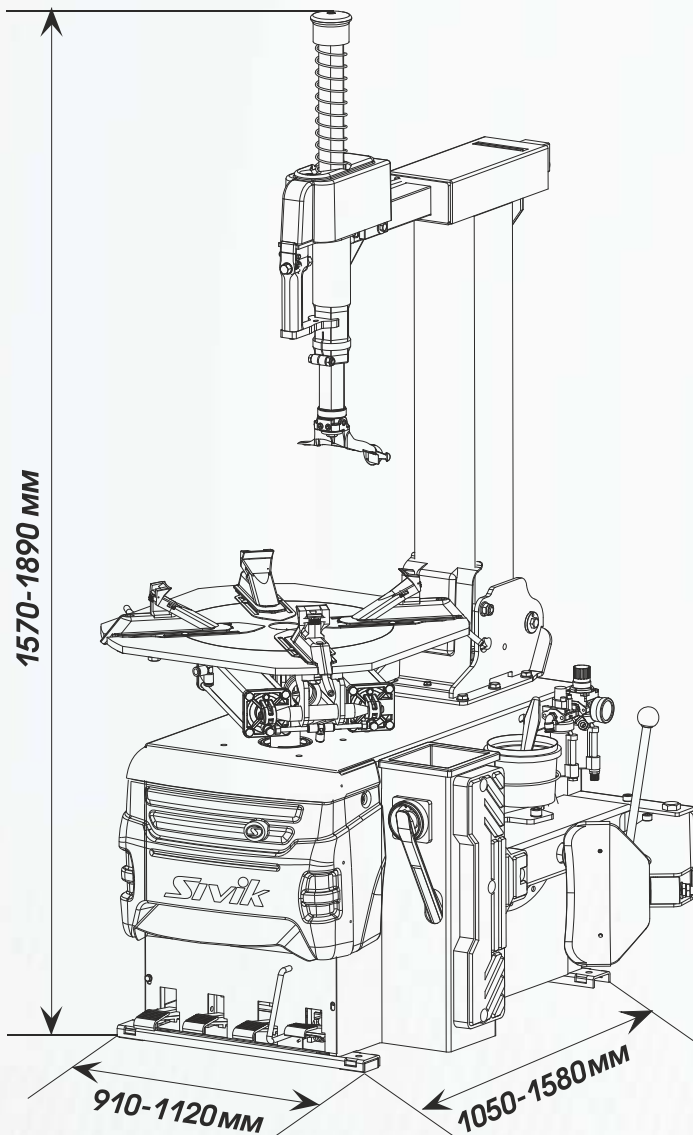
Рисунок 4 Установка стенда
